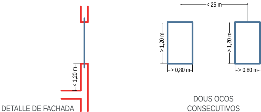
DETALLE DE FACHADA
